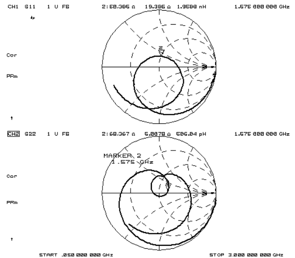
Zin, Zout
