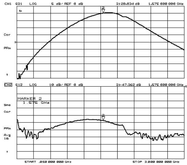
S21, S12
