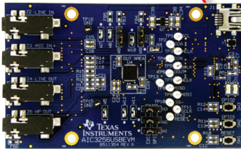
TLV320AIC3256USB EVM
